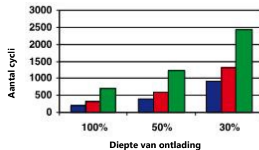
Grafiek 2: Levensduur bij cyclisch gebruik
