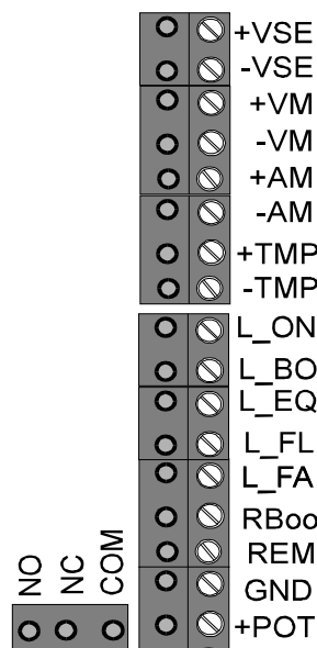
Figuur 8. Positie van de externe aansluitingen.
