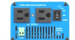
Phoenix omvormer 12/180 met Nema 5-15R stopcontacten
