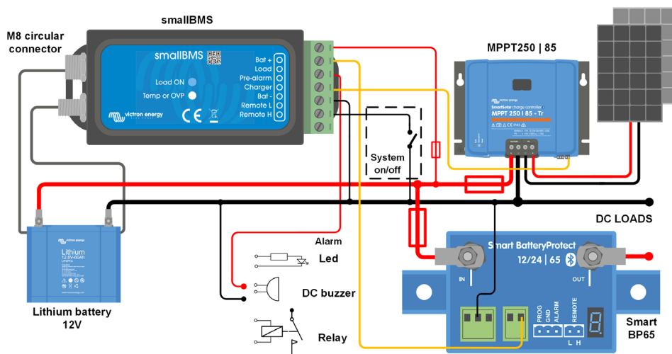
Afbeelding 1: Toepassingsvoorbeeld voor een DC niet net gekoppelde systeem, met systeem aan-/uitschakelaar tussen L en accu-negatief
