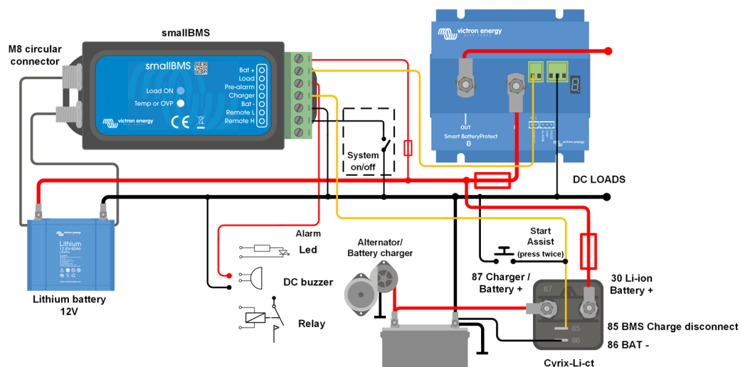
Afbeelding 2: Toepassingsvoorbeeld voor een voertuig of boot, met systeem aan-/uitschakelaar tussen L en accu-negatief
